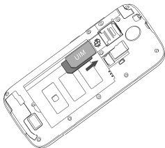
图 4 安装 UIM/SIM 卡
